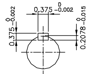
INPUT SHAFT
