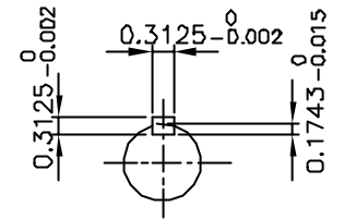
INPUT SHAFT
