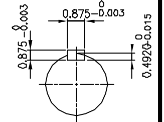
INPUT SHAFT
