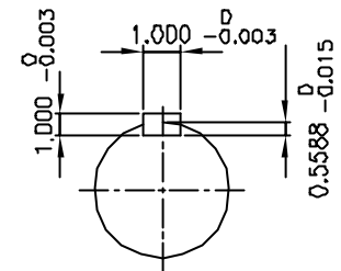
INPUT SHAFT
