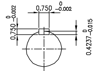
INPUT SHAFT
