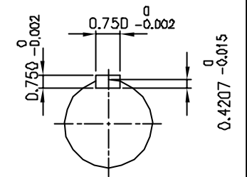
INPUT SHAFT
