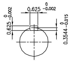
INPUT SHAFT
