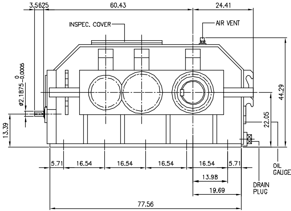
INPUT SHAFT
