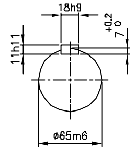
INPUT SHAFT
